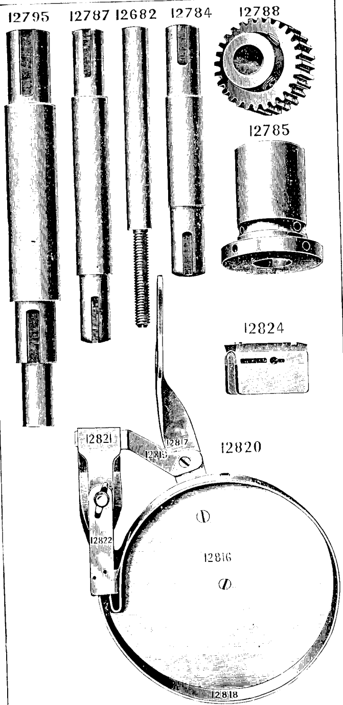
PLATE 1075—ONE-HALF SIZE
