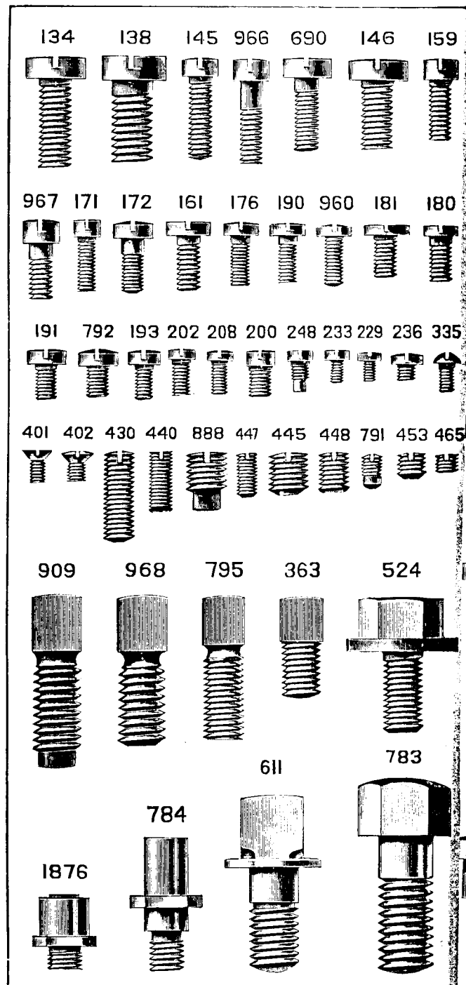
PLATE 1058—FULL SIZE
